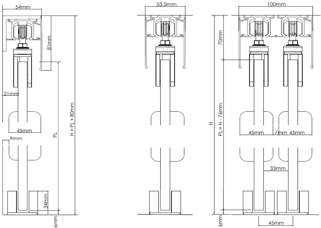
WANDMONTIERTE EINZELTÜR ODER DOPPELTÜR
