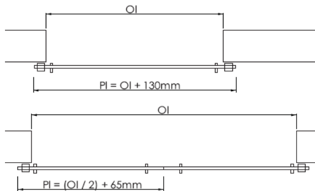
DECKENMONTIERTE EINZELTÜR ODER DOPPELTÜR
